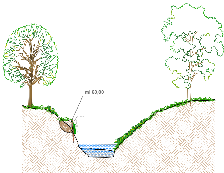
sezione C-C POST INTERVENTO
