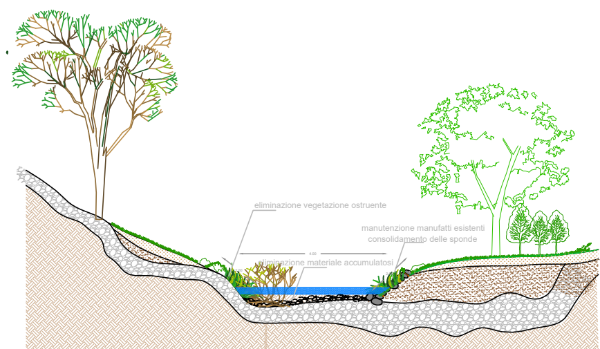
sezione B-B ANTE INTERVENTO
