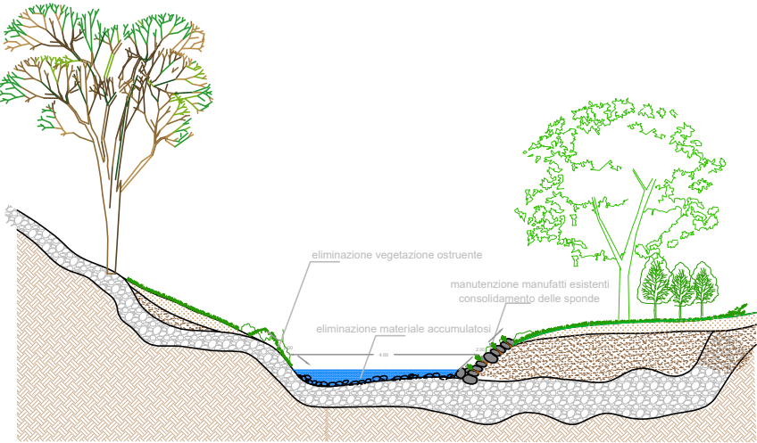
sezione B-B POST INTERVENTO
