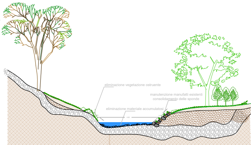
sezione B-B POST INTERVENTO
