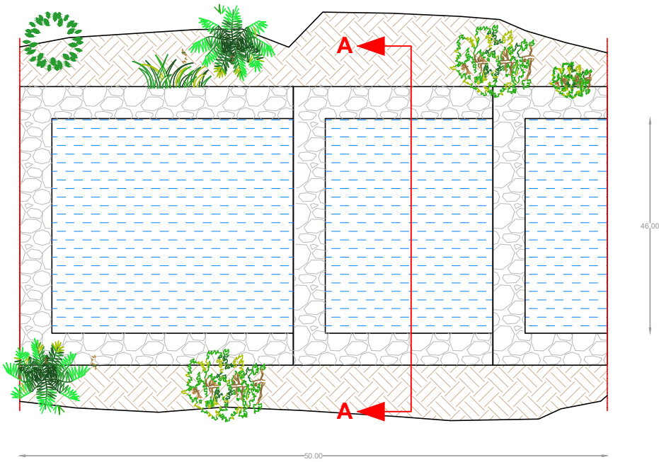
pianta POST INTERVENTO
