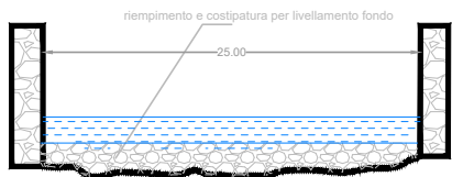
sezione AA POST INTERVENTO
