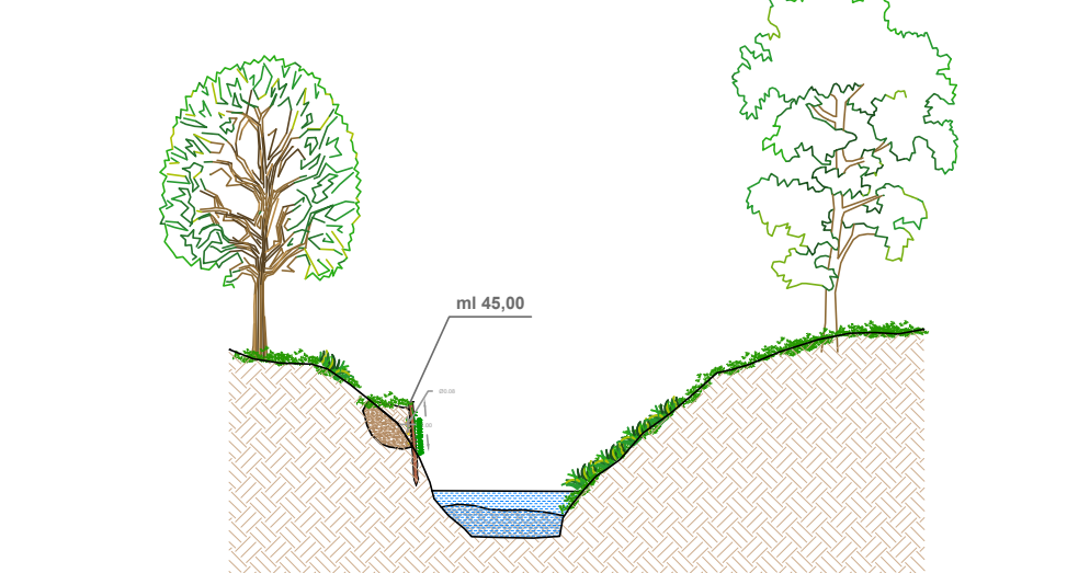
sezione C-C POST INTERVENTO
