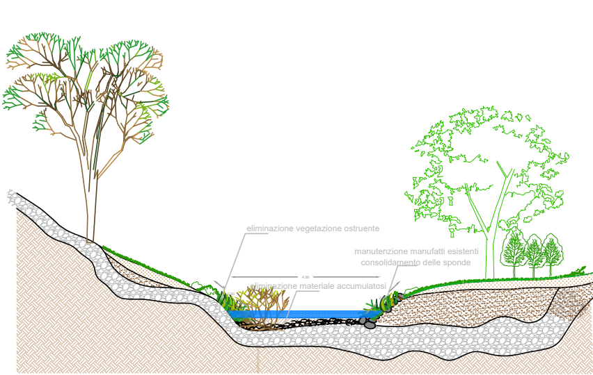
sezione B-B ANTE INTERVENTO
