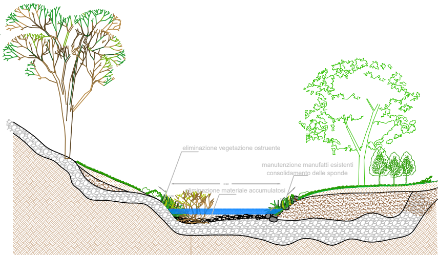
sezione B-B ANTE INTERVENTO
