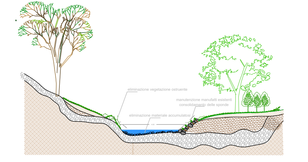
sezione B-B POST INTERVENTO
