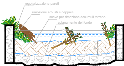
sezione AA ANTE INTERVENTO
