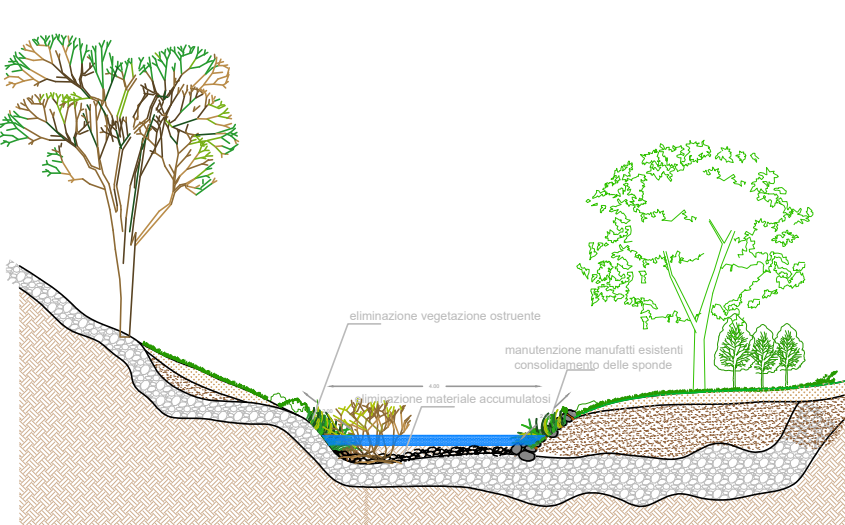
sezione B-B ANTE INTERVENTO
