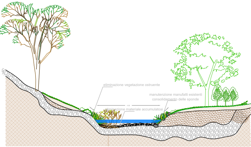
sezione B-B ANTE INTERVENTO
