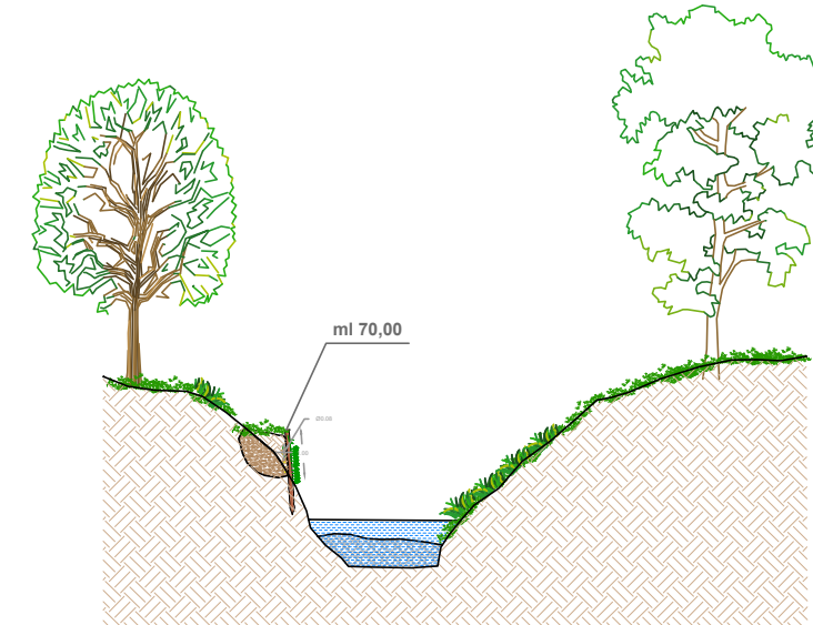
sezione C-C POST INTERVENTO
