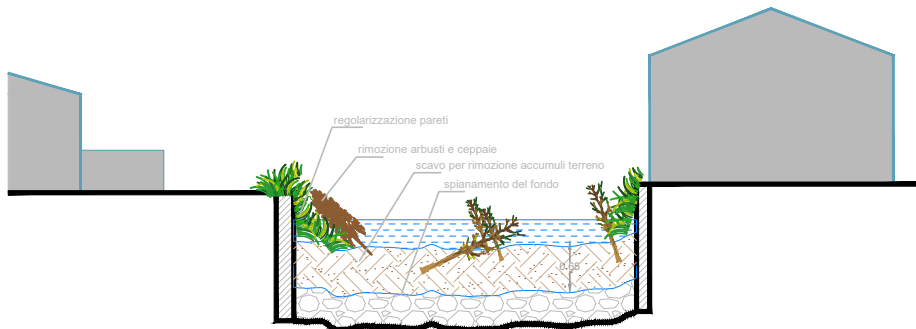
sezione AA ANTE INTERVENTO
