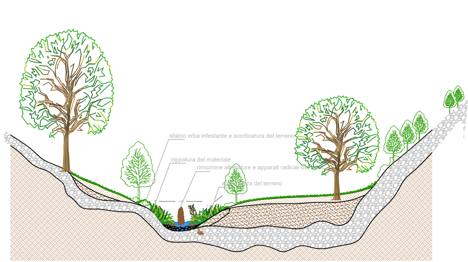
sezione A-A ANTE INTERVENTO
