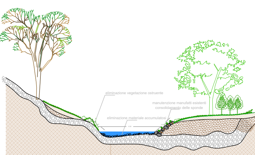
sezione B-B POST INTERVENTO
