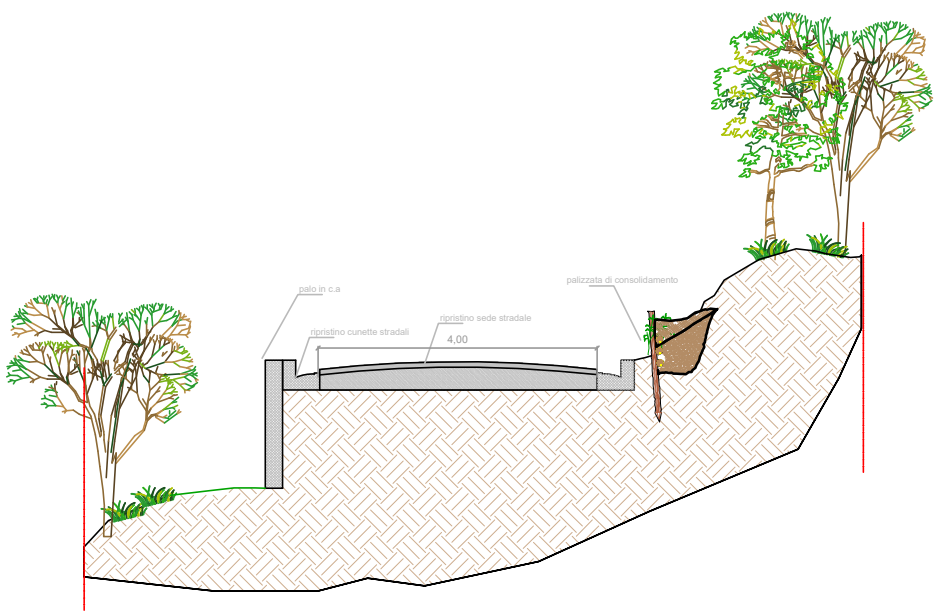
sezione AA POST INTERVENTO
