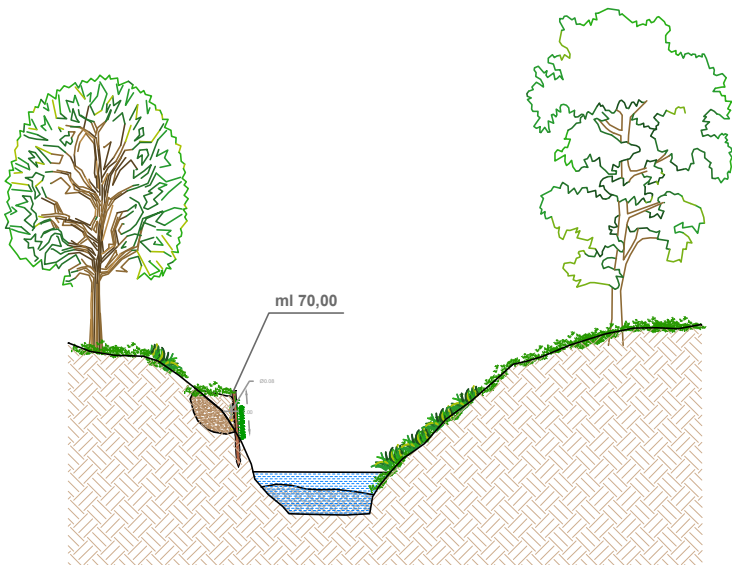
sezione C-C POST INTERVENTO
