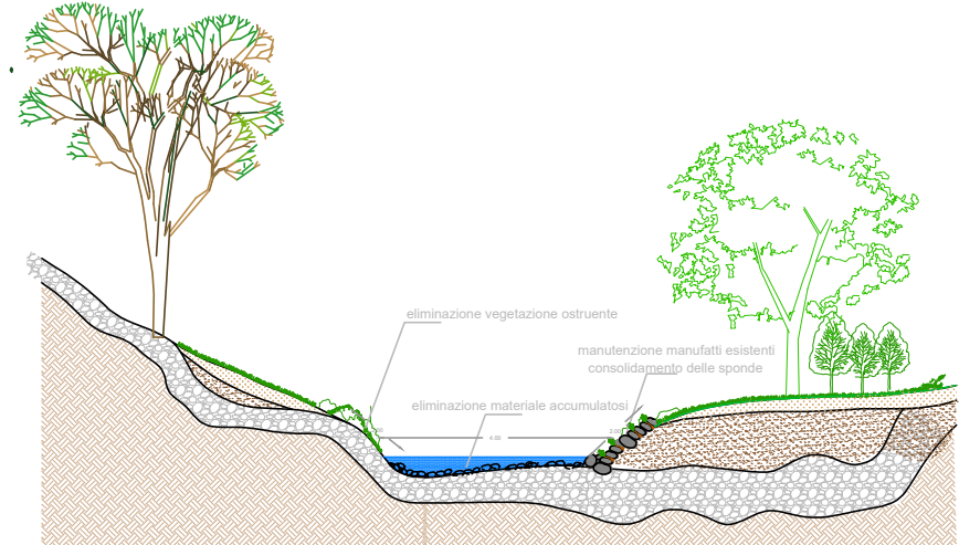
sezione B-B POST INTERVENTO
