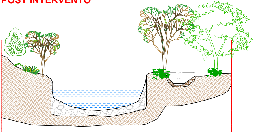
sezione tipo POST INTERVENTO
