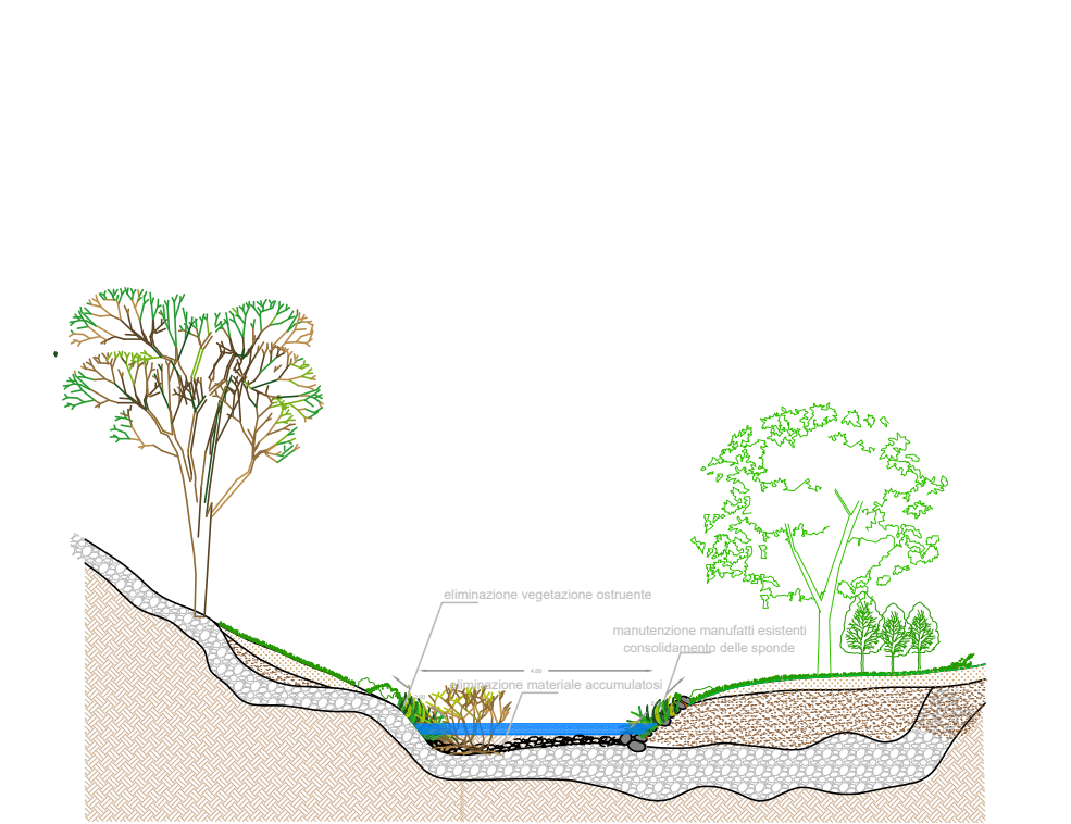
sezione B-B ANTE INTERVENTO
