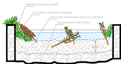
sezione AA ANTE INTERVENTO
