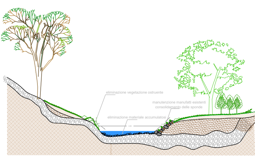
sezione B-B POST INTERVENTO
