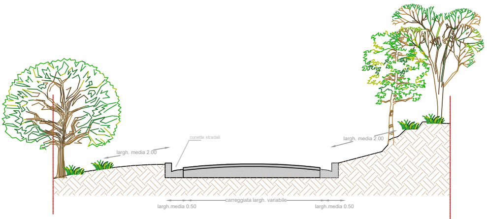
sezione AA POST INTERVENTO
