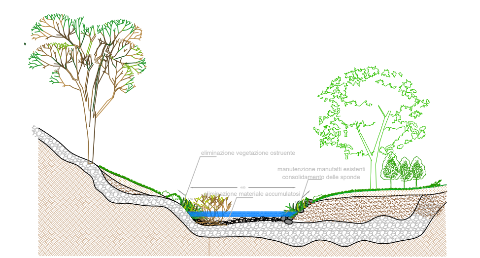
sezione B-B ANTE INTERVENTO
