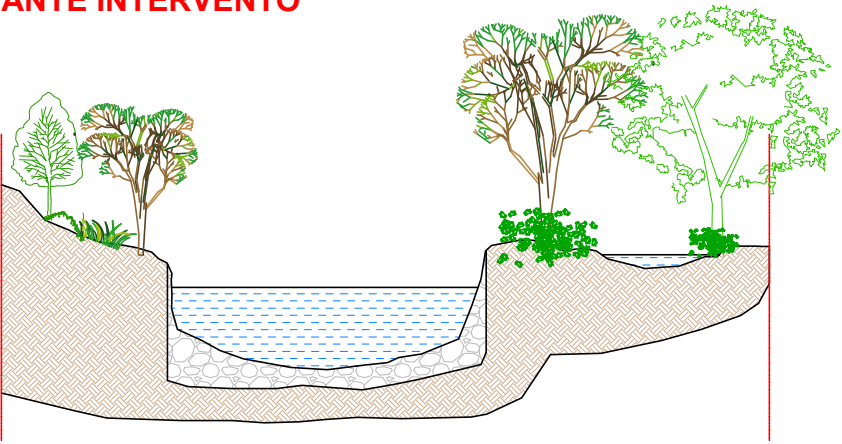
sezione tipo ANTE INTERVENTO
