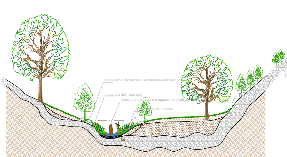
sezione A-A ANTE INTERVENTO
