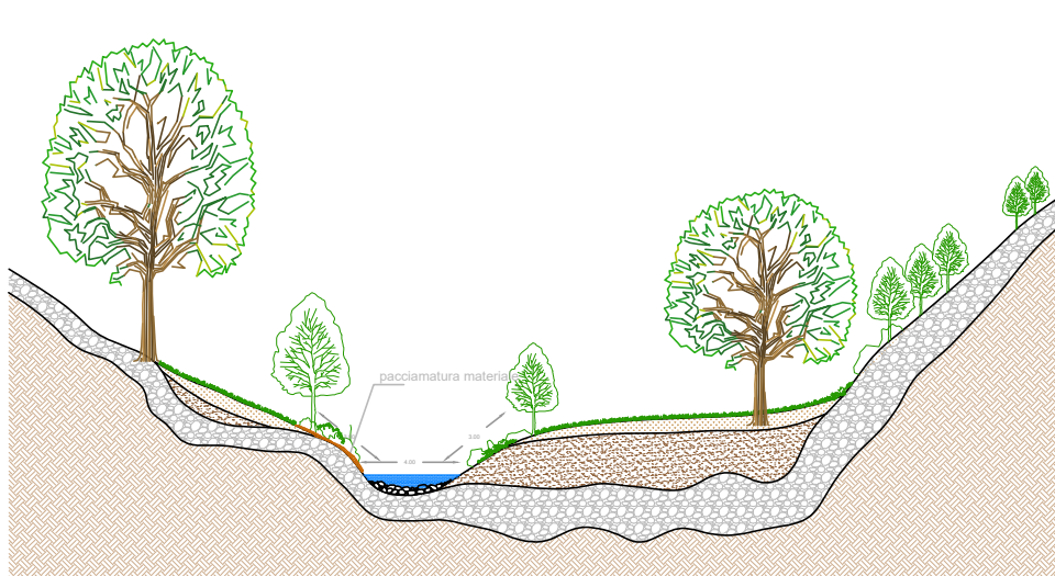
sezione A-A POST INTERVENTO
